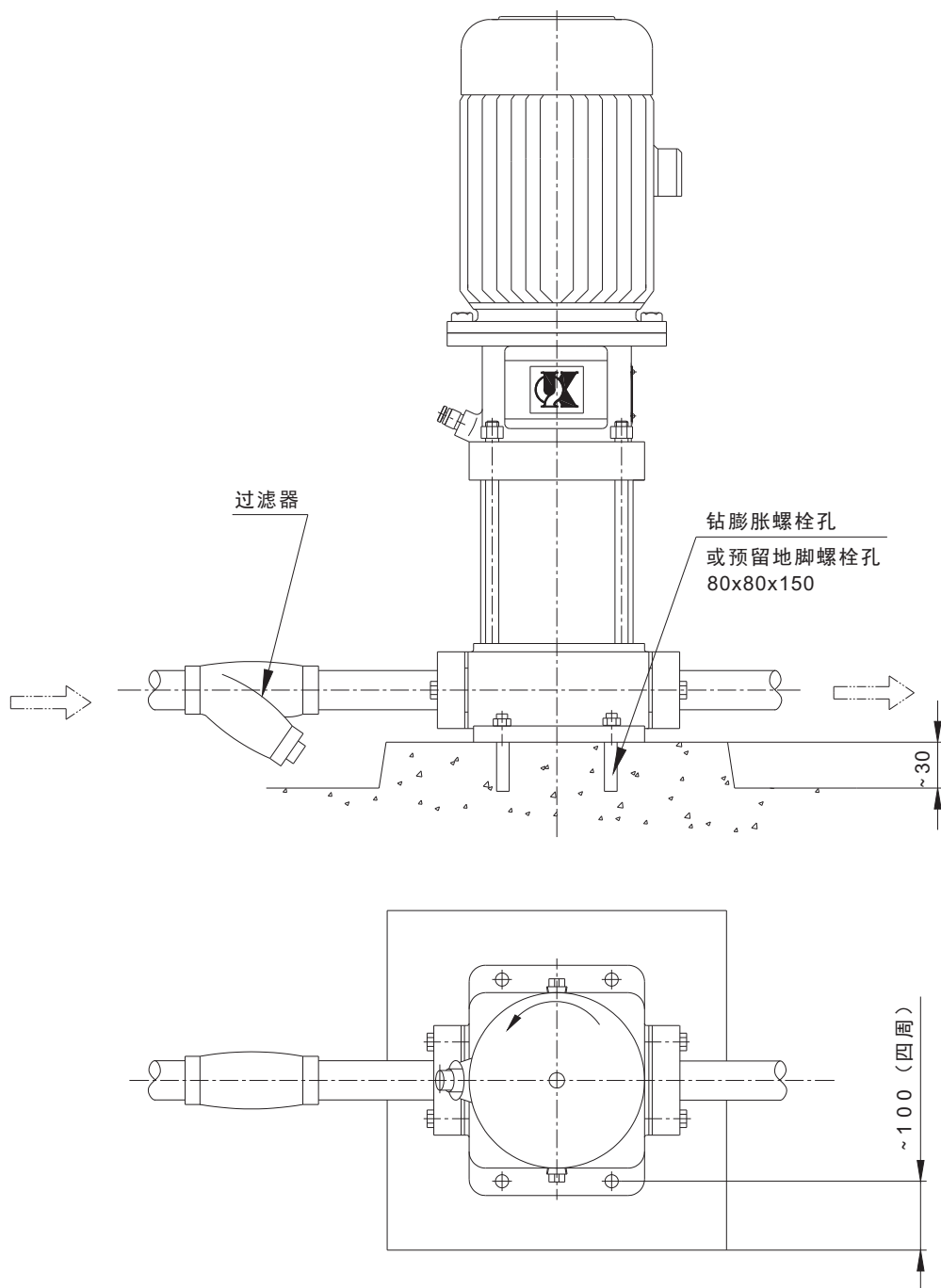
KQDP、KQDQ 安装图
