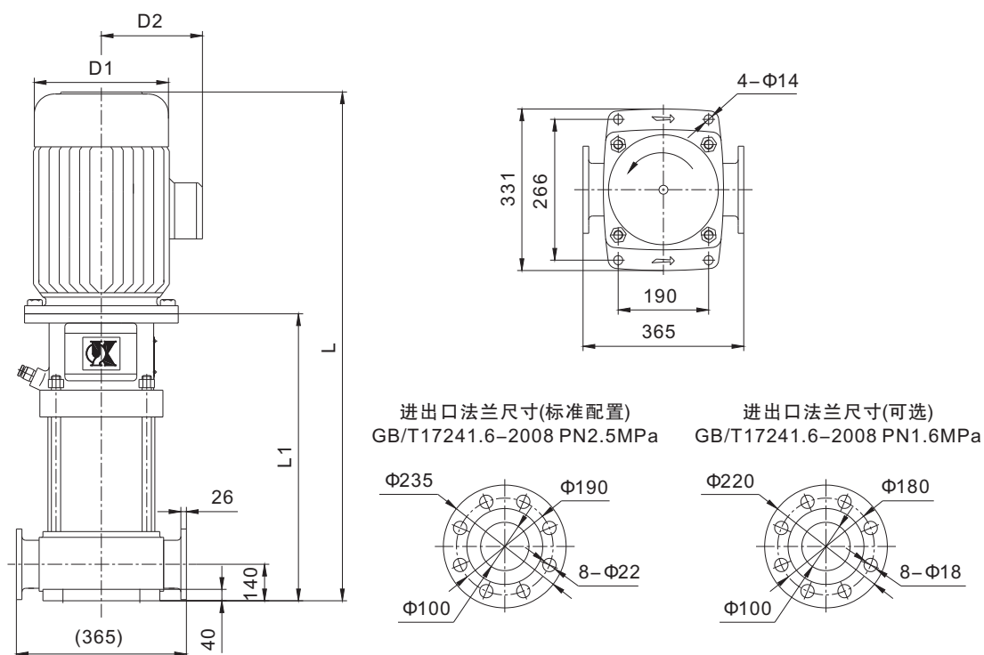
安装图
