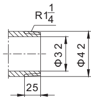
进出口螺纹联接尺寸(可选)
