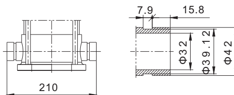
进出口卡口联接尺寸(可选)
