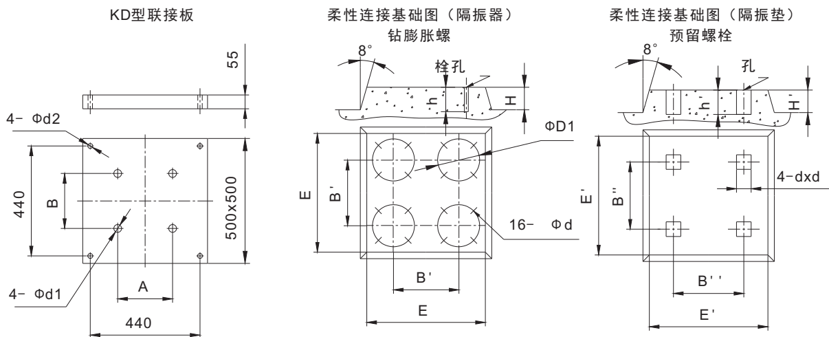
柔性安装基础尺寸图
