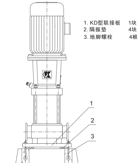
柔性连接（隔振垫）
