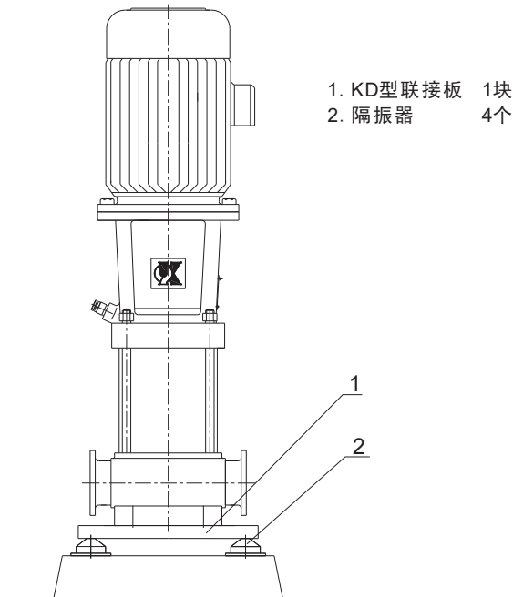
柔性连接（隔振器）
