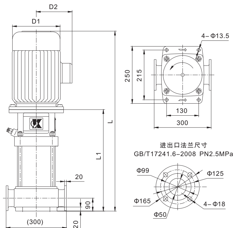
安装图
