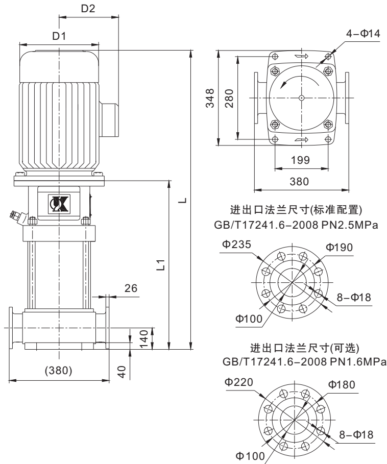
安装图
